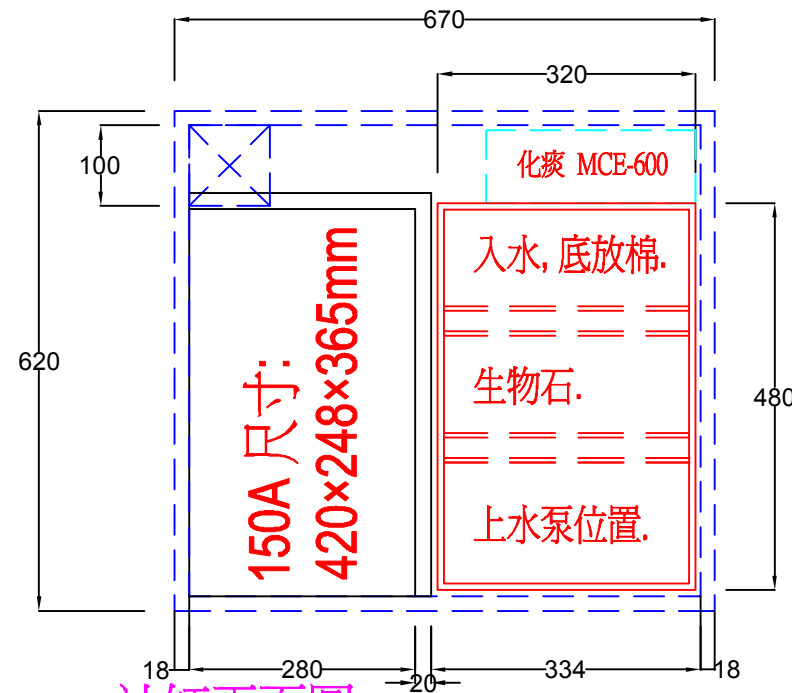
沙缸平面圖.
