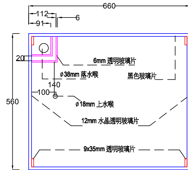
主缸平面圖.
