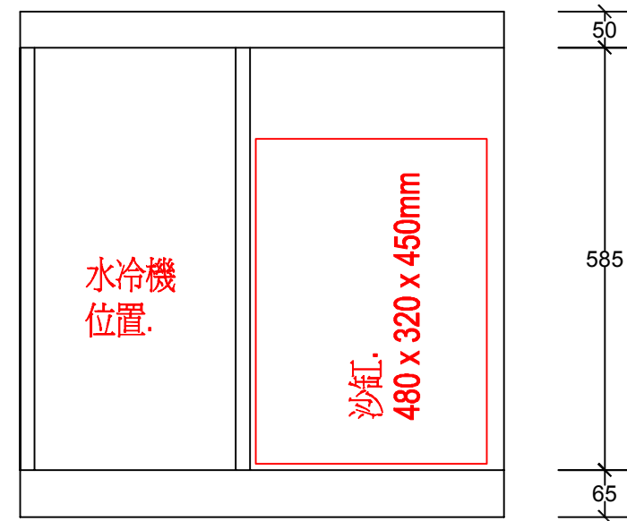
沙缸立面圖.
